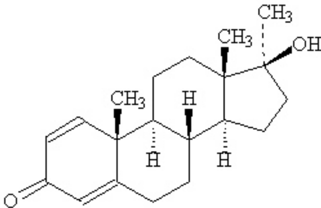
Methandrostenolone (Dianabol)
