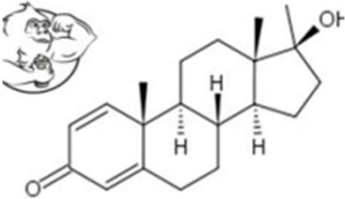
Methandrostenolone (Dianabol)
